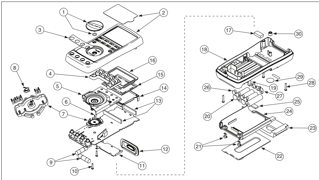
图 12.更换零件
