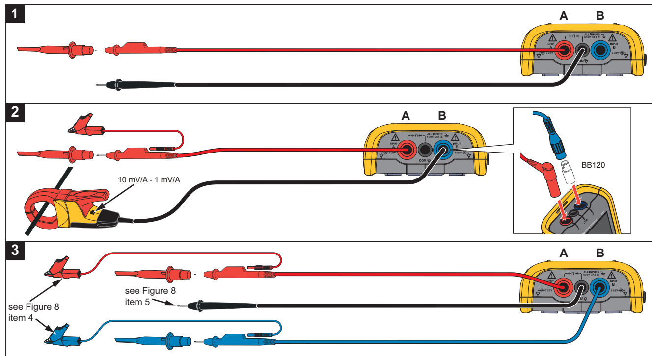
图 7. 测量设置
